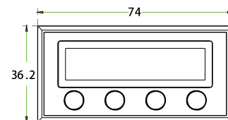
正视图 Front view
