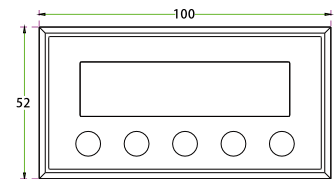
正视图 Front view
