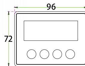
正视图 Front view
