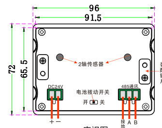
底视图 Bottom view
